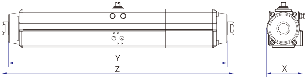
尺寸表 Length of pneumatic actuator
