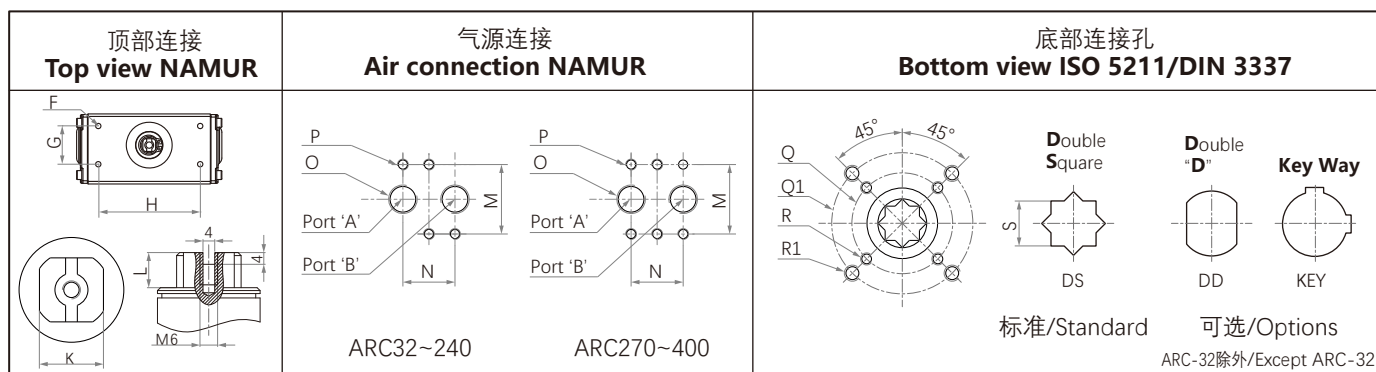
连接尺寸图 Connection
