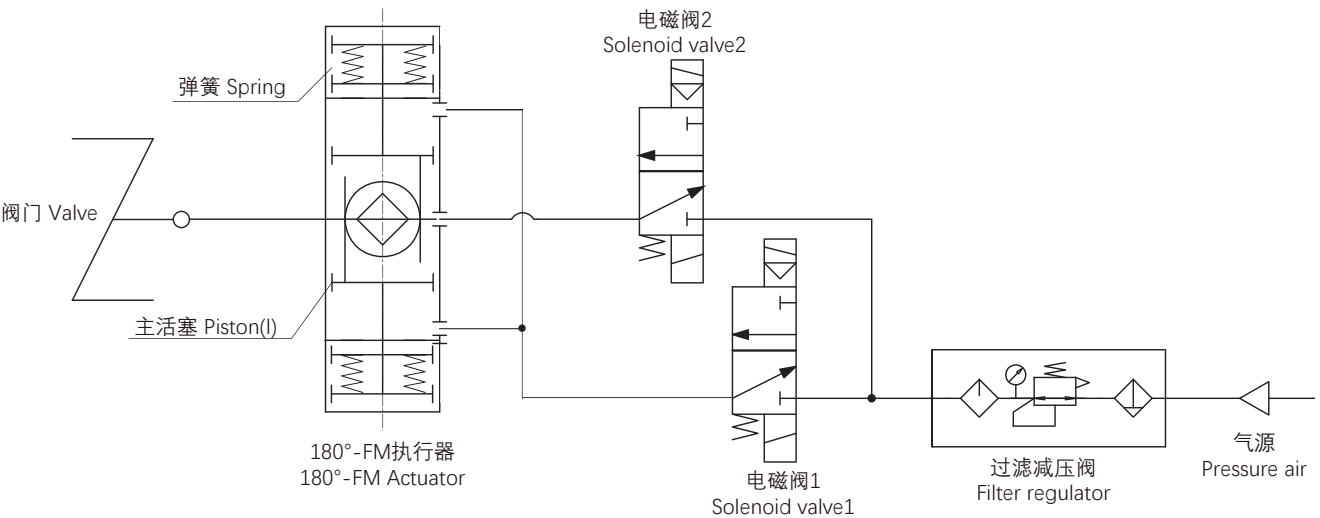
工作原理图 Schematic Diagram
